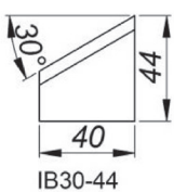
30° Outil de coupe chanfrein interne, Hauteur 44 mm [IB30/44] Référence: NOZ-000023
