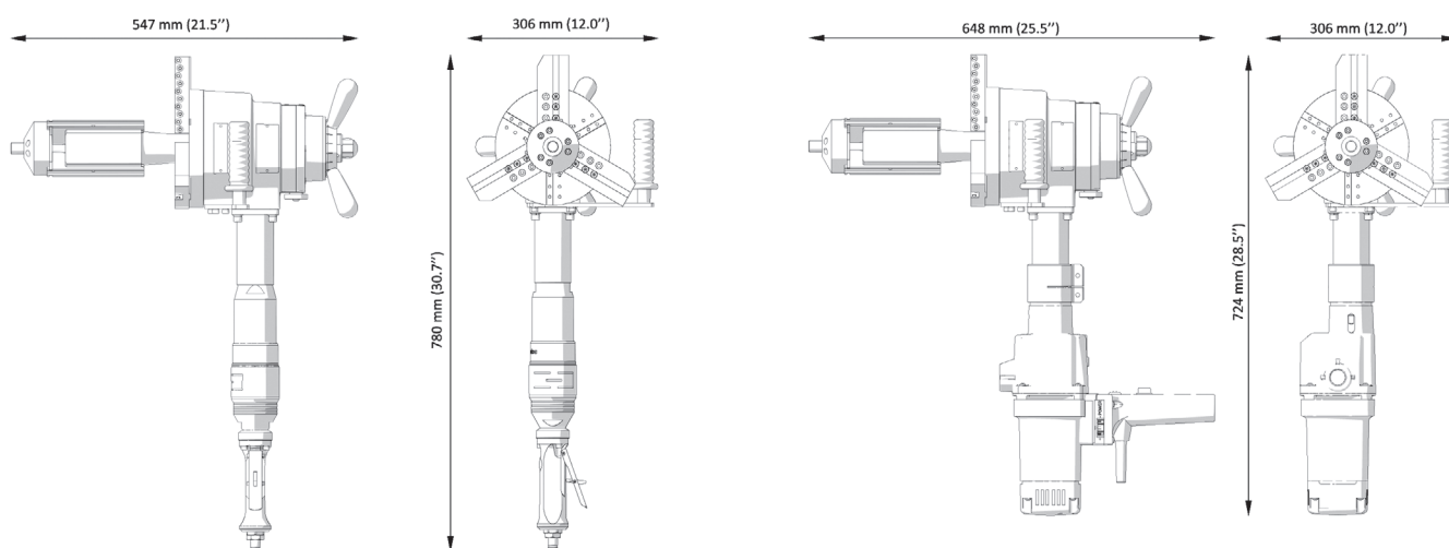
PRO-10 PB avec moteur pneumatique
