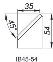
45° Outil de coupe chanfrein interne, Hauteur 54 mm [IB45/54] Référence: NOZ-000026
