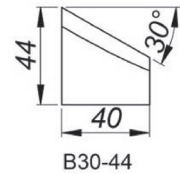
30° Outils de coupe chanfrein, Hauteur 44 mm [B30/44] Référence: NOZ-000018
