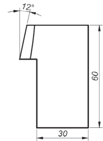
12° Outil de coupe special, Hau- teur 60 mm Référence: NOZ-000086
