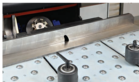
Accès facile à la tête de coupe et aux plaquettes
