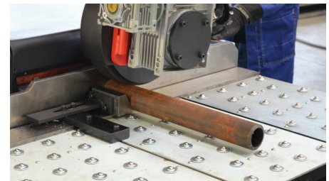
Possibilité de chanfreiner des tubes (extérieur)
